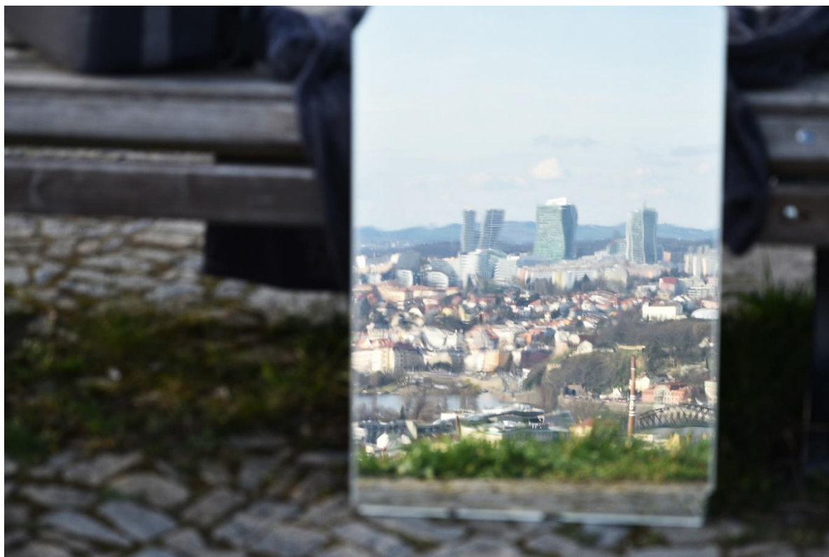
Obrázek 3. Křivé zrcadlo.
